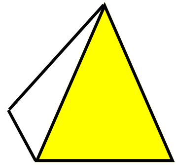
pyramid
