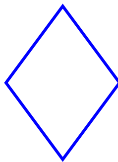
rhombos
